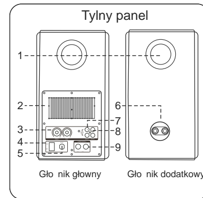
Głośnik główny
